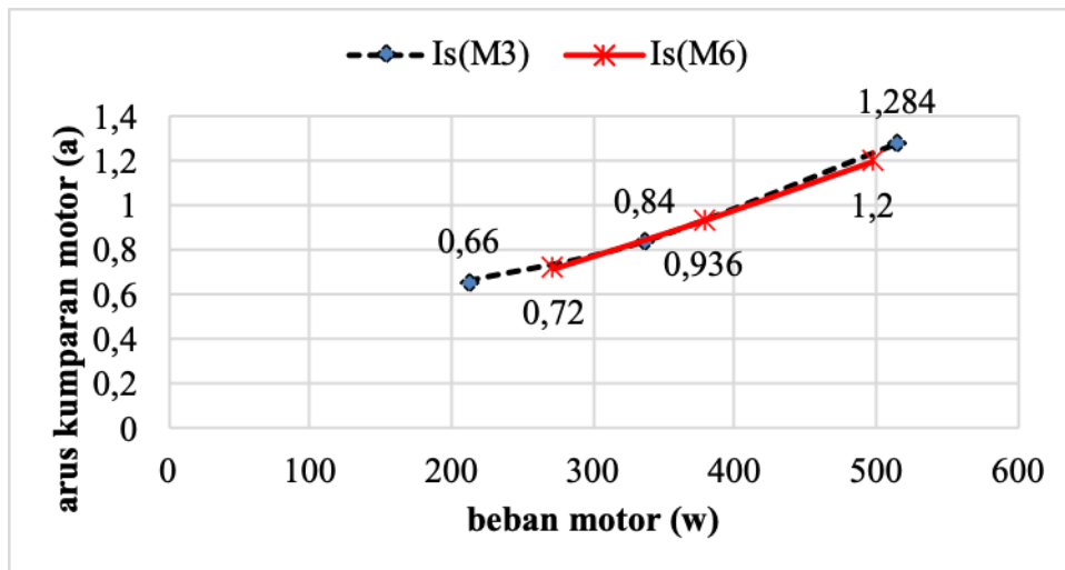
Gambar 2 Perbandingan grafik Arus motor induksi 3 fasa konvensional dan motor desain 6 fasa 6 medan fluks 1 lapis kumparan simetris.
