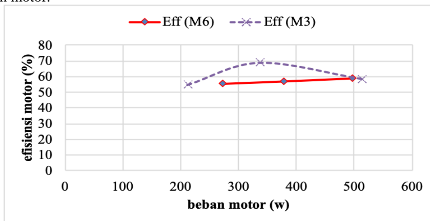
Gambar 1 Perbandingan grafik efisiensi motor induksi 3 fasa konvensional dengan motor desain 6 fasa 6 medan fluks 1 lapis kumparan simetris.
