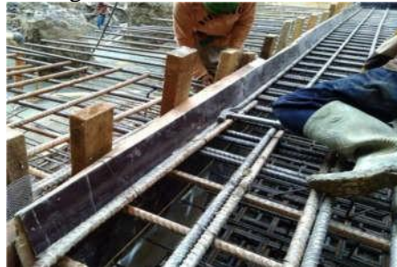
Gambar 3 Pekerjaan Bekisting
