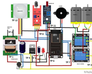
Gambar 11. Titik Pengukuran Rangkaian
