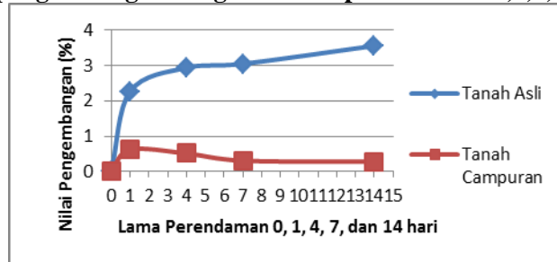
Grafik hasil pengembangan dengan variasi perendaman 0,1,4,7, dan 14 hari
