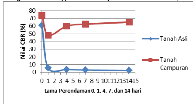
Grafik hasil uji CBR dengan variasi perendaman 0,1,4,7 dan 14 hari
